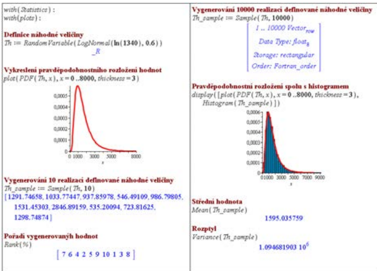
Obrázek 5.45: Práce s balíkem Statistics .
